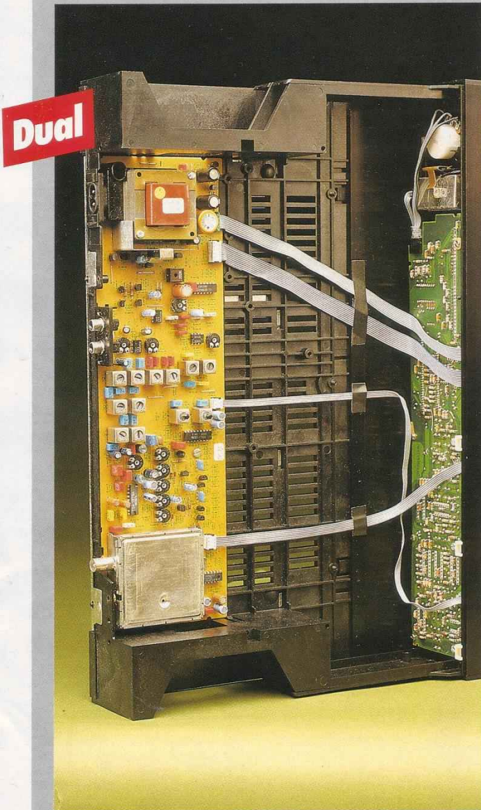
Da verschlägt's einem den Atem: Spitzenqualität aus so wenig Elektronik! Die Steuerplatine rechts ist in SMD-Technik bestückt
